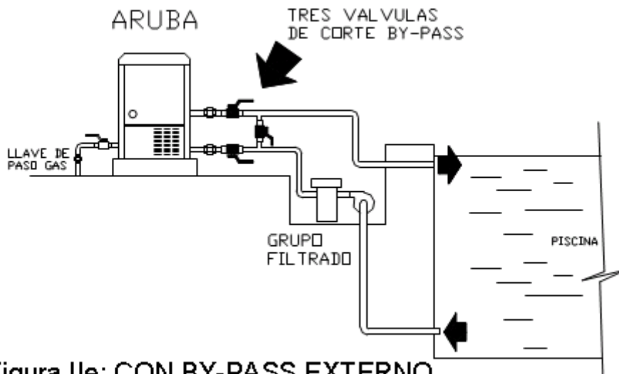
Figura 11e: CON BY-PASS EXTERNO
