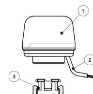
1) Attuator elettrotermico 2) Cavo elettrico 3) Aggancio rapido
