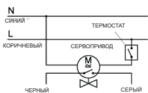
ЭЛЕКТРИЧЕСКАЯ СХЕМА 4-Х ПРОВОДНОГО СЕРВОПРИВОДА С МИКРОВЫКЛЮЧАТЕЛЕМ ART. 979-982
