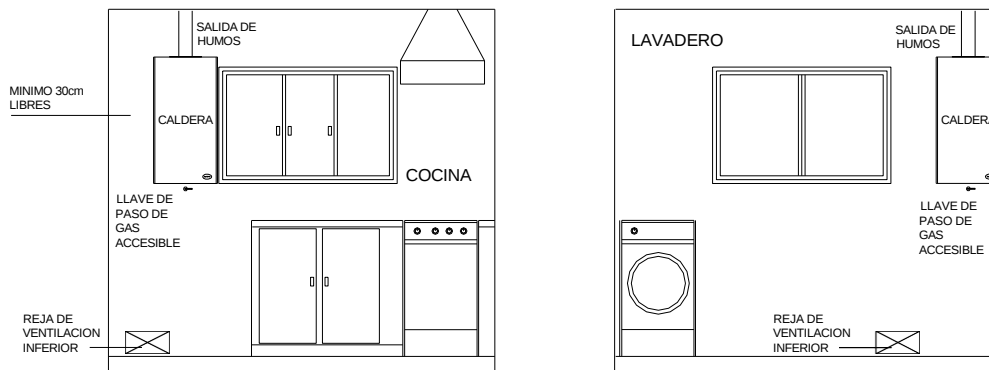
Figura II i - Esquema instalación de caldera mural dentro de la cocina o de un lavadero
