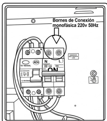
Conexión eléctrica caldera Monofásica 220V 50Hz ~
