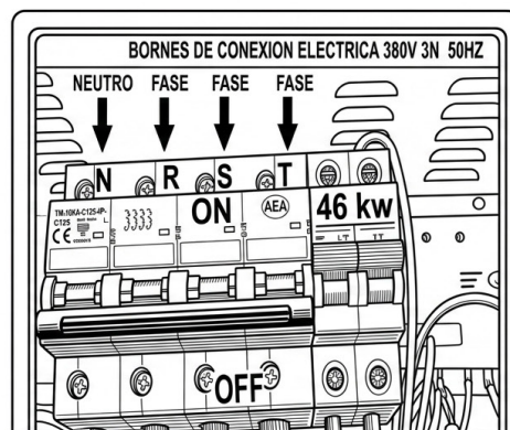
Conexión eléctrica caldera Trifásica 380V 3N~ 50Hz
